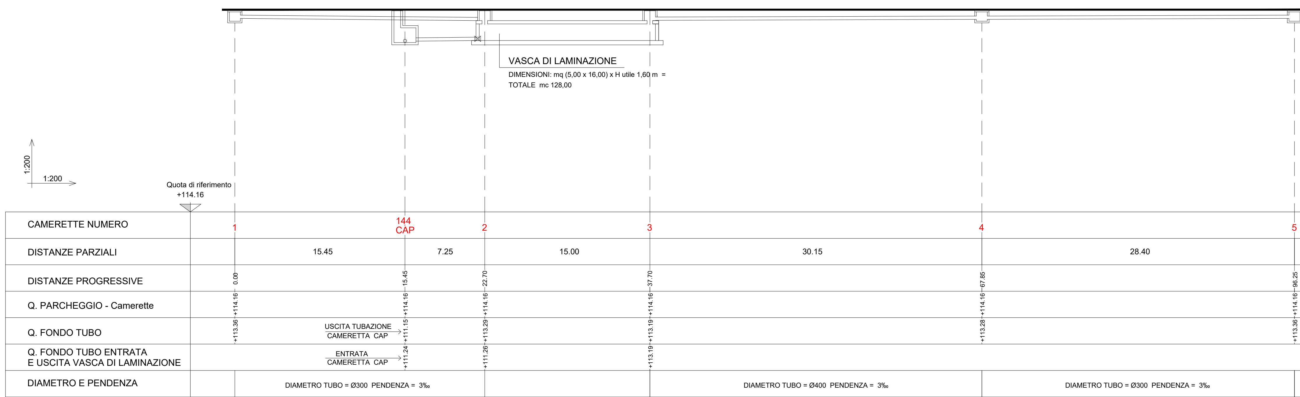
PROFILO LONGITUDINALE
